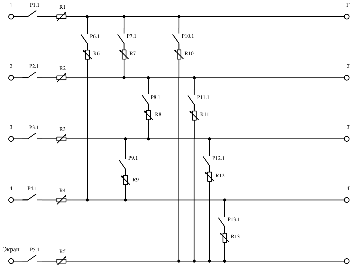
Рис. 3. Принципиальная схема исполнительной части устройства внесения неисправностей в электрический кабель связи
